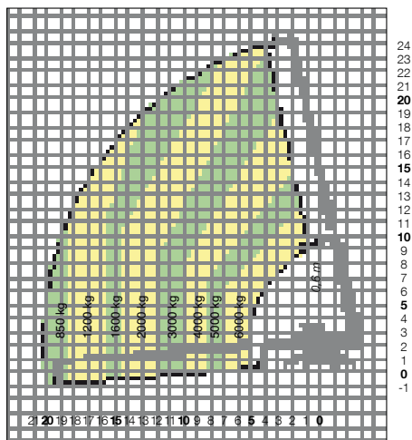
ROTO 60.24 MCSS MIT LASTGABELN AUF ABSTÜTZUNGEN - 360°
