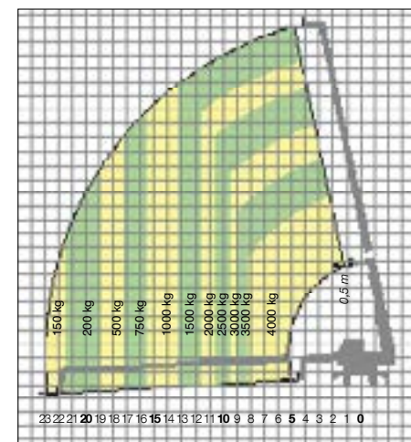
ROTO 40.26 MCSS MIT LASTGABELN AUF ABSTÜTZUNGEN - 360°
