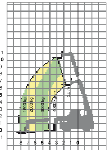
ROTO 50.10 S MIT LASTGABELN AUF REIFEN
