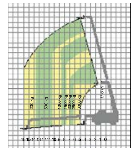
ROTO 45.21 MIT LASTGABELN AUF REIFEN
