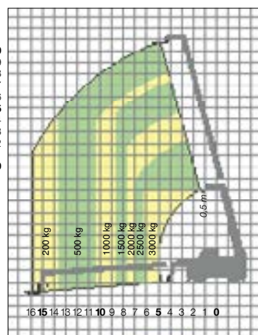
ROTO 45.21 MCSS MIT LASTGABELN AUF REIFEN
