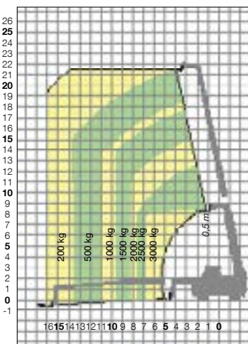
ROTO 40.26 MCSS MIT LASTGABELN AUF REIFEN
