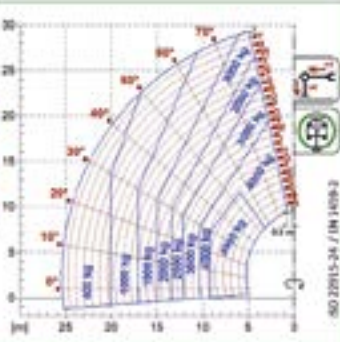
ROTO50.30
