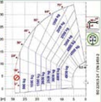
ROTO50.35
