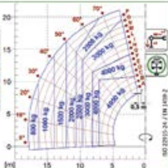
ROTO50.21
