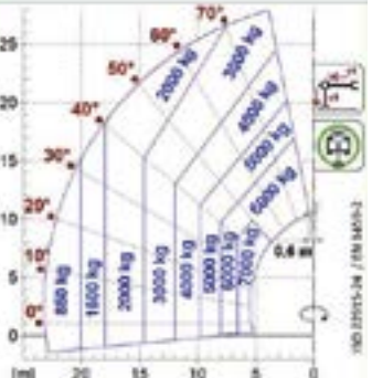
ROTO70.28
