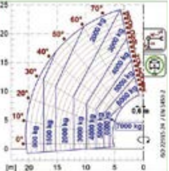
ROTO70.24
