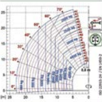
ROTO50.26
