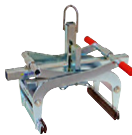
TRITTSCHWELLENVERSETZZANGE PROBST TSZ-UNI
