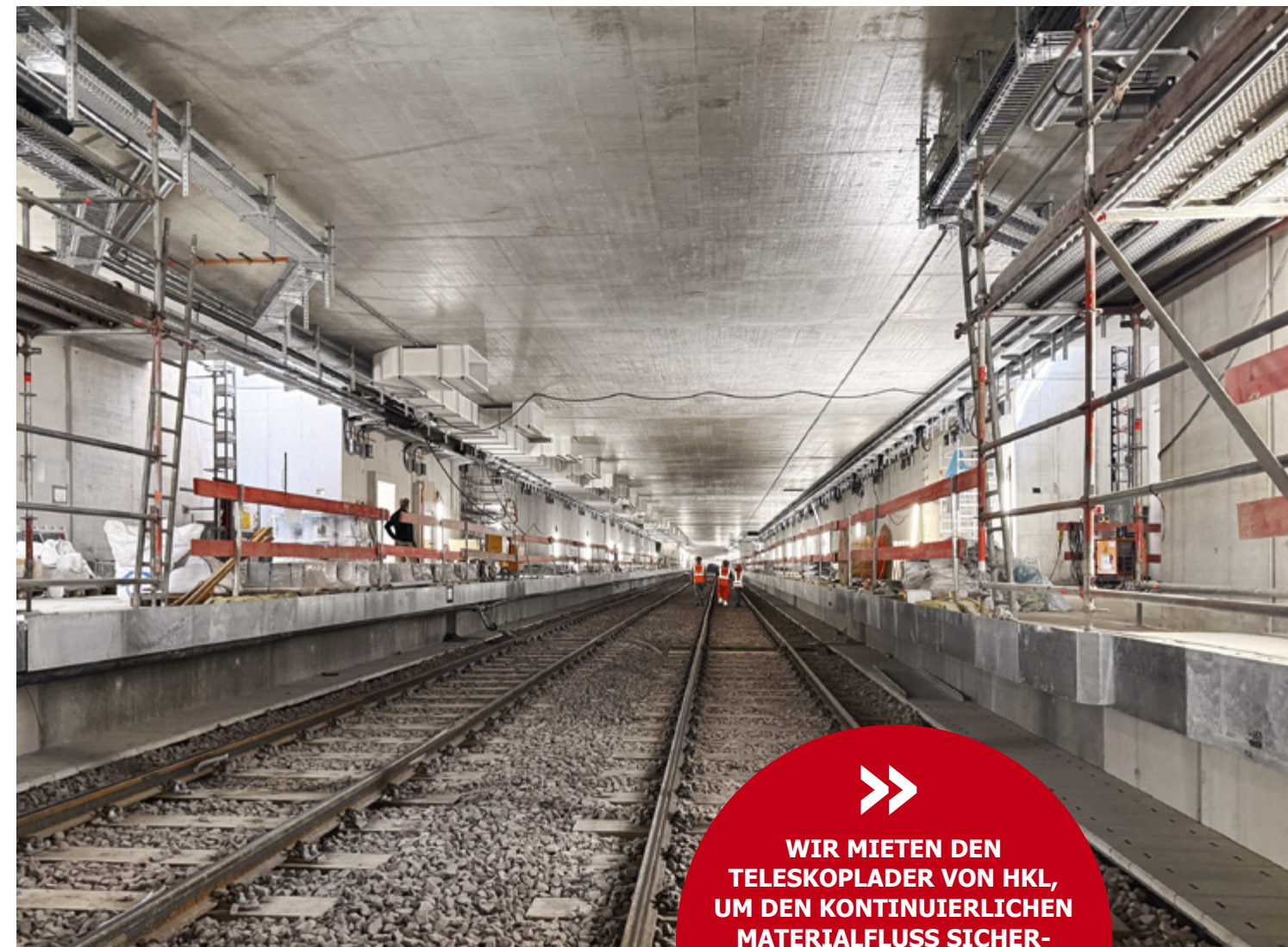
Der größte Teil des Rohbaus der Teilstrecke zwischen den Haltestellen Stollenstraße und Horner Geest ist weitgehend fertiggestellt, Schwellen und Schienen sind hier bereits verlegt.
